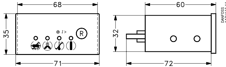
Indication module IMR for TI 180 E and TI 630 E
