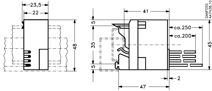
Indication module IMR for TI 180 E and TI 630 E
