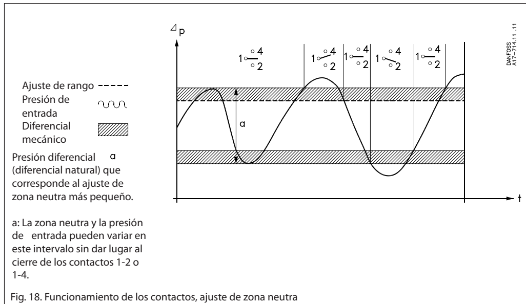
Fig. 18. Funcionamiento de los contactos, ajuste de zona neutra
